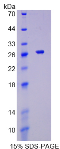
15% SDS-PAGE
