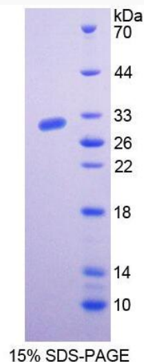
15% SDS-PAGE
