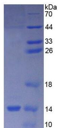
15% SDS-PAGE
