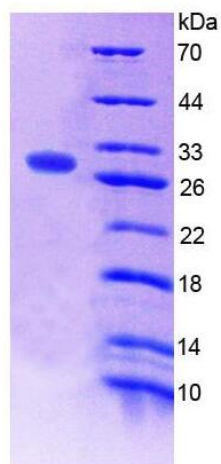
15% SDS-PAGE
