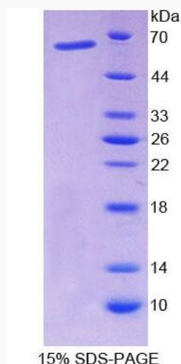
15% SDS-PAGE
