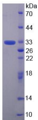
15% SDS-PAGE
