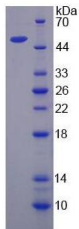
15% SDS-PAGE
