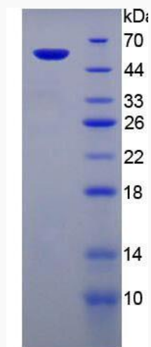
15% SDS-PAGE
