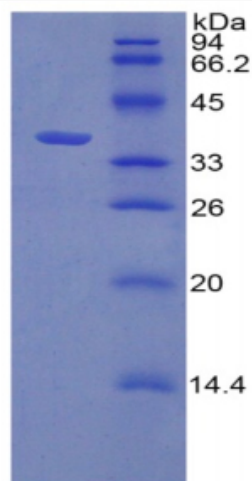
15% SDS-PAGE
