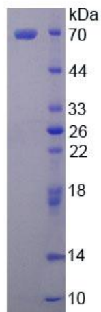
15% SDS-PAGE
