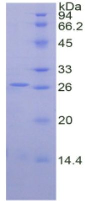
15% SDS-PAGE
