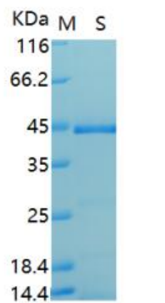
SDS-PAGE Result
