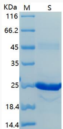
SDS-PAGE Result
