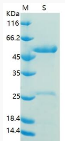
SDS-PAGE Result
