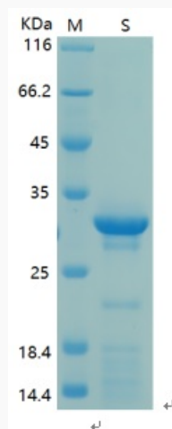
SDS-PAGE Result
