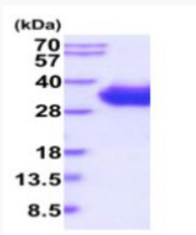
15% SDS-PAGE(3ug)
