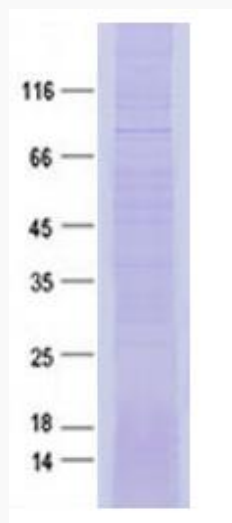
SDS-PAGE
