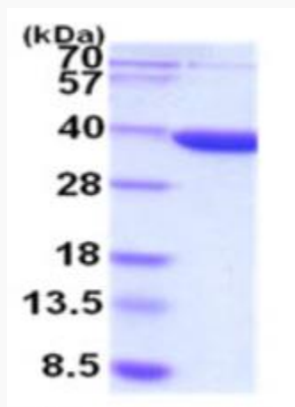
15% SDS-PAGE(3ug)
