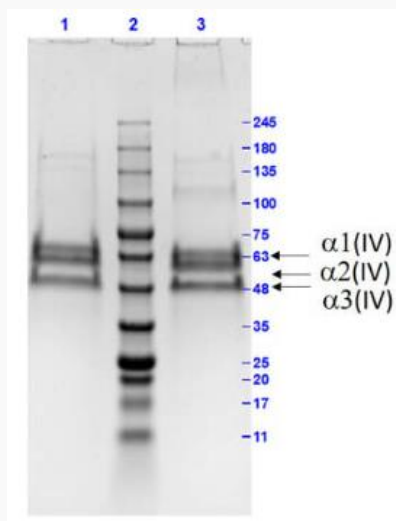
SDS-PAGE
