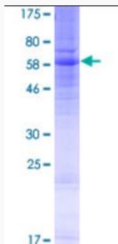
SDS-PAGE
