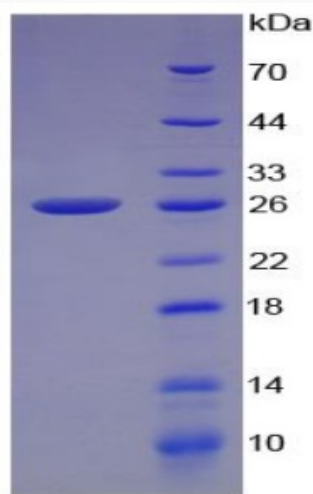
15% SDS-PAGE
