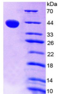
15% SDS-PAGE
